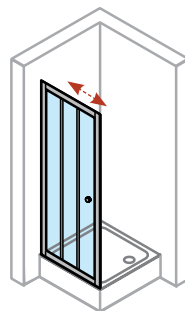
Posuvné sprchové dvere 2-dielne s pevným segmentom GT2 FS, pre montáž vľavo alebo vpravo
