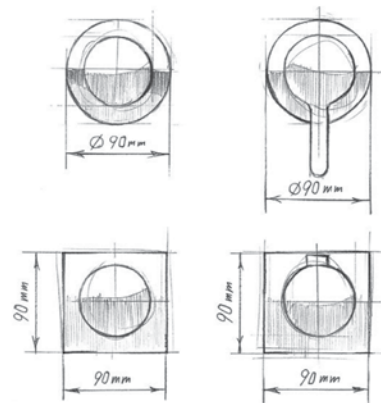
prepínací a uzatvárací ventil s prípojkou a držiakom hadice, chróm, (pre použitie s termostatickou/pákovou batériou, hlavovou sprchou, ručnou sprchou)
