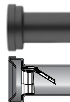
Trubka WC DN90 s klapkou proti hľadavcom dĺžka 180 mm
